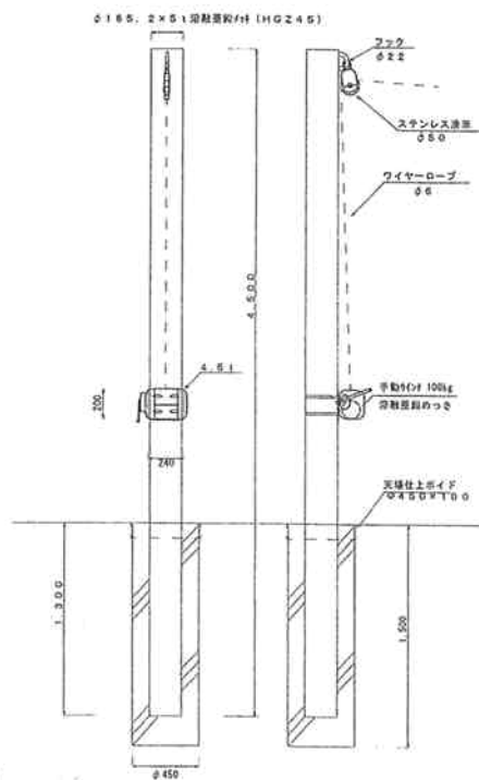
2(t)-支柱詳細図 S=1/20
