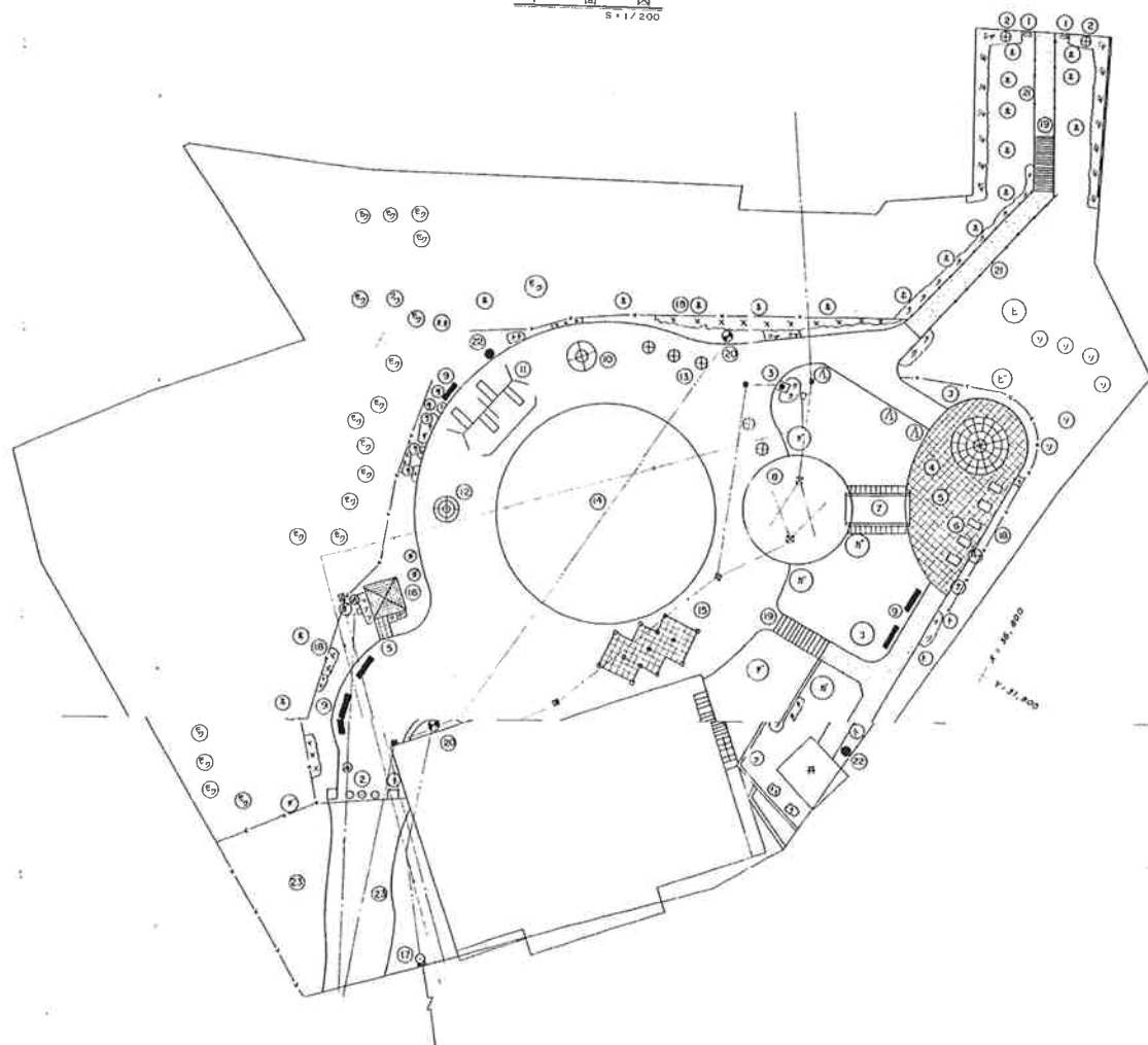
平面図 S=1/200
